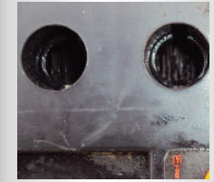
BAJO NIVEL DE ELECTROLITO Provocado por sobrecargas y/o aplicación incorrecta.
