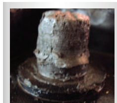
FALDONEADO Sucede al golpear la terminal cuando no está bien abierta.
