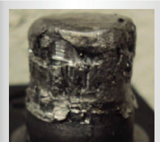
APRETADO Por utilizar terminales inadecuadas o usar terminal negativa en poste positivo.
