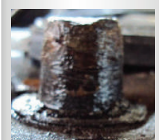
HUNDIDO Por golpes directos al poste o tornillo.
