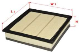
Filtro AIRE A-65530
