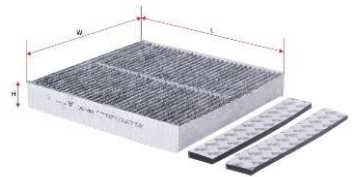
Filtro AIRE CABINA * con carbón activado CAC-1801
